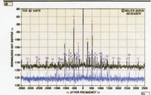
ROTEL RSP-1098 AV PROCESSOR: JITTER WITH 48kHz & 96kHz LPCM DIGITAL INPUTS
