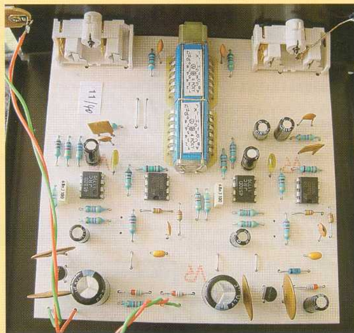
En redig design i all sin enkelhet på ett enkelsidigt kretskort. Såväl diskreta komponenter som IC i signalvägen.
